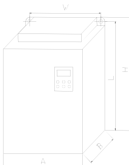
图 2-1-A 外形尺寸及安装尺寸示意图
