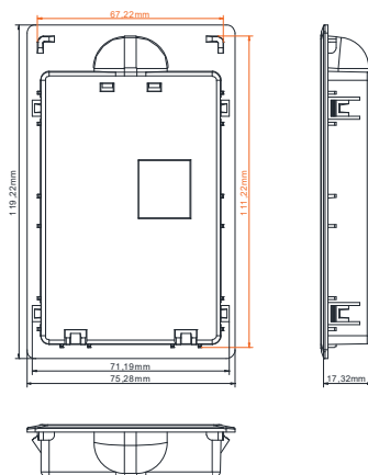
图 2-1-B 外引面板托架外形尺寸及安装尺寸示意图
