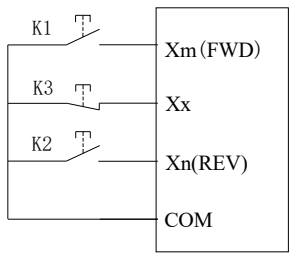
三线式控制模式 1 示意图
